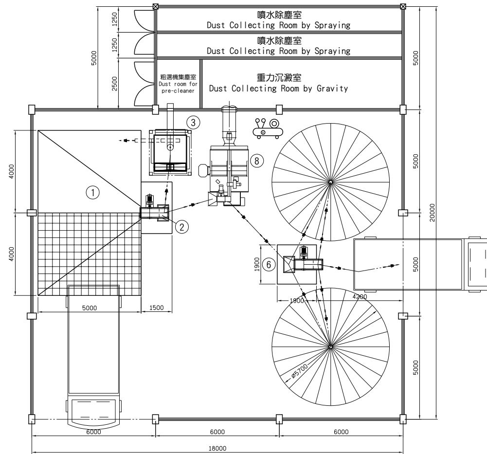
乾燥機上視圖 Top view
