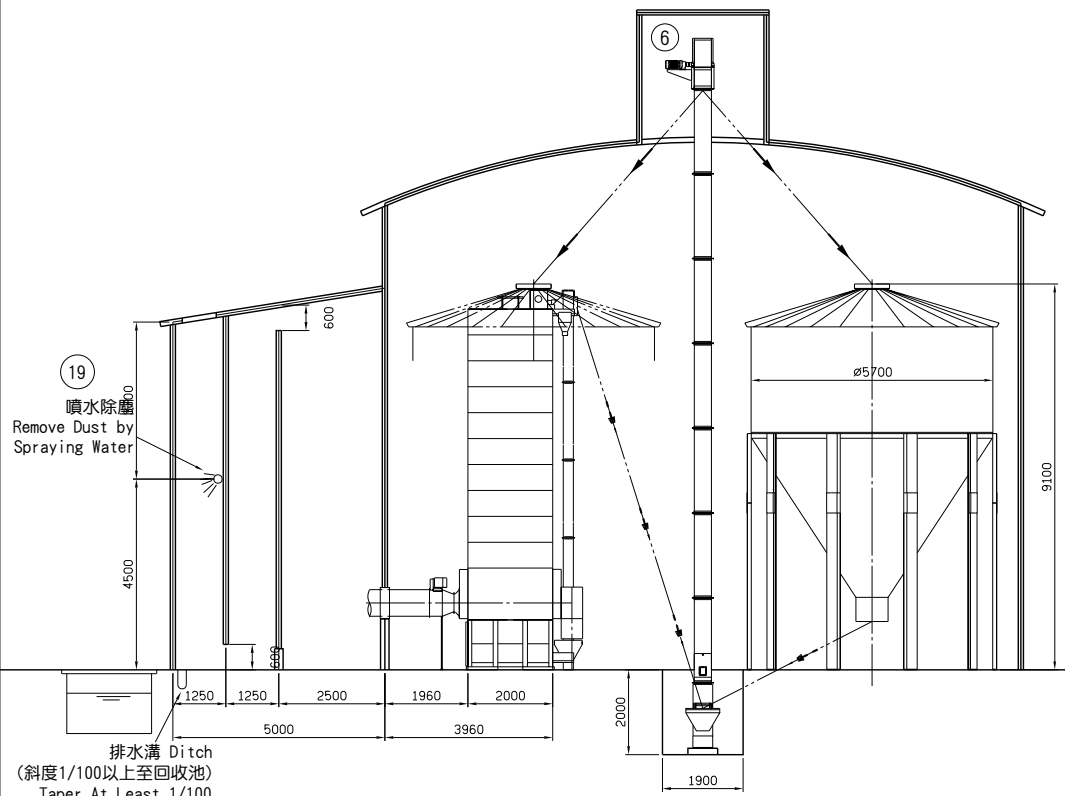
乾燥機側視圖 Side view
